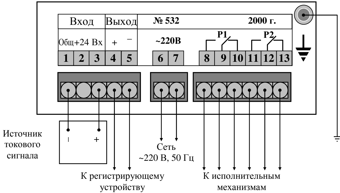
Рисунок Б.3 - Пример подключения источника с токовым выходным сигналом к ПКЦ-1101.05 или ПКЦ-1101.42
