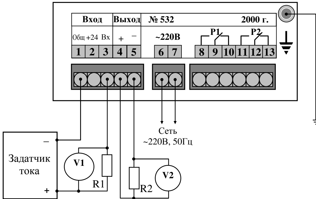
Рисунок В.1 - Схема внешних соединений при калибровке и настройке ПКЦ-1101.05 или ПКЦ-1101.42
