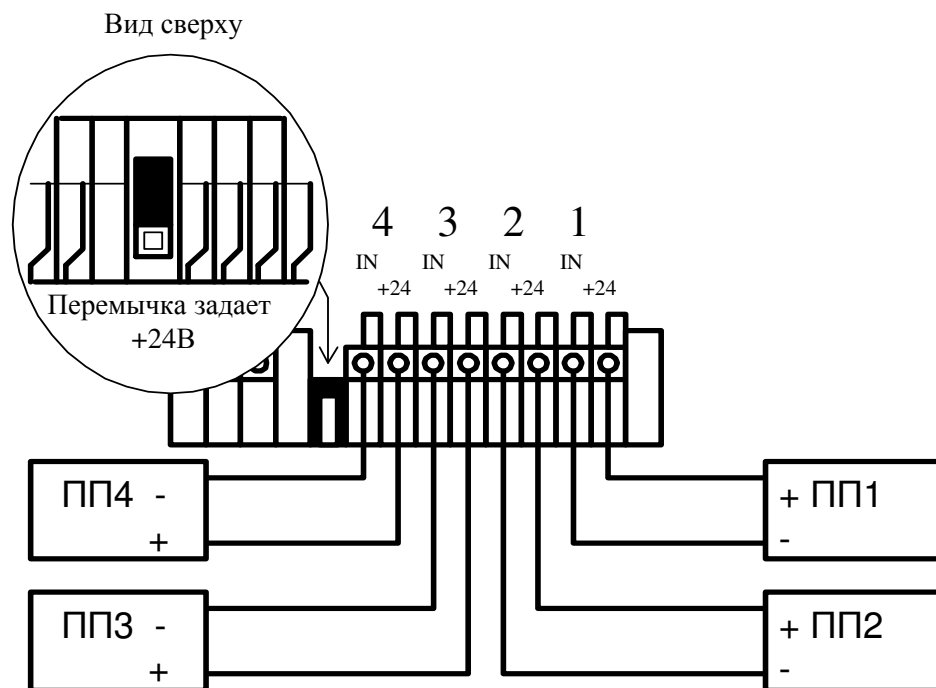
Рисунок 4 - Пример подключения пассивных первичных преобразователей
