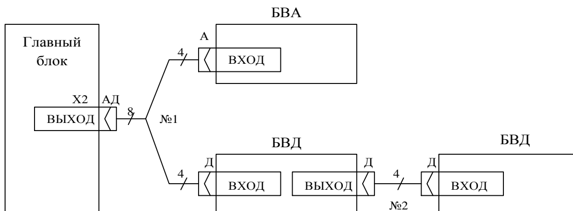
Рисунок 2 - Схема межблочных соединений ПКЦ-12К
