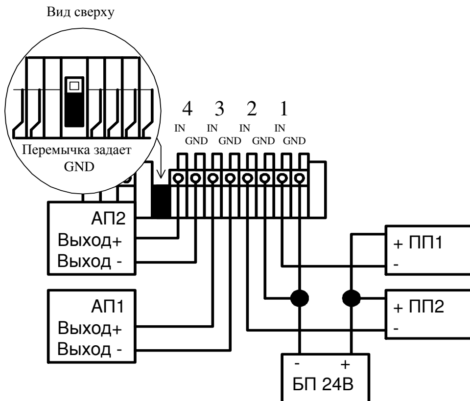
Рисунок 5 - Пример подключения активных первичных преобразователей (АП1, АП2) и пассивных первичных преобразователей (ПП1, ПП2) с внешним блоком питания БП
