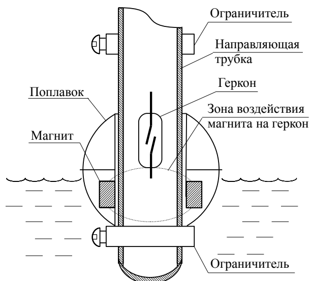
Рисунок С.3 - Реализация замыкающего (NO) контакта
